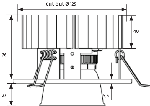
Abmessungen Aura Aperius R und Aura Aperius C
