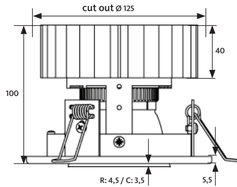
Abmessungen Aura Aperius SR
